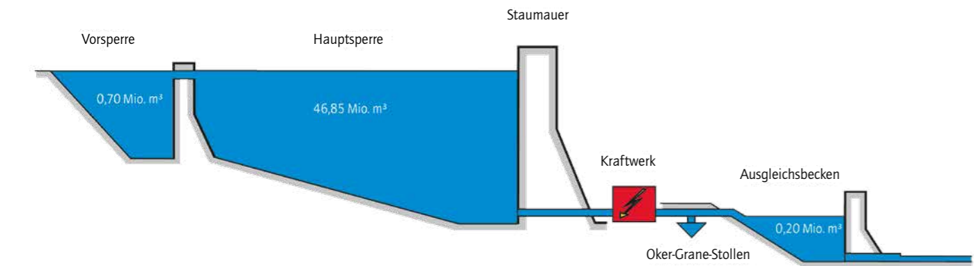
System der Okertalsperre
